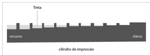
Sistema rotogravura
